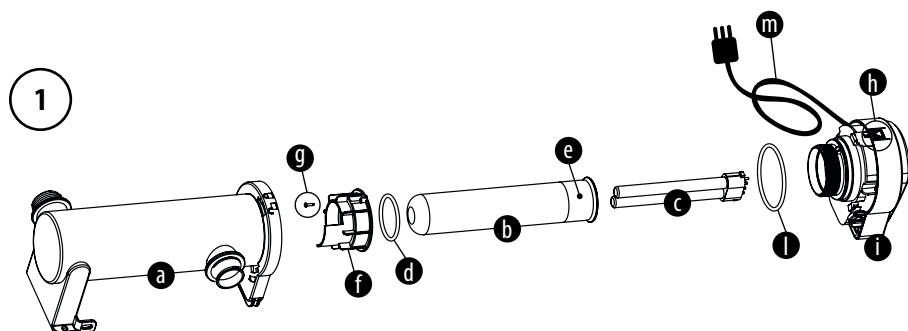
Fig. 1 Denominazione dei componenti • Name of components Dénomination des composants • Bezeichnung der Bestandteile Naam van de componenten • Наименование компонентов
